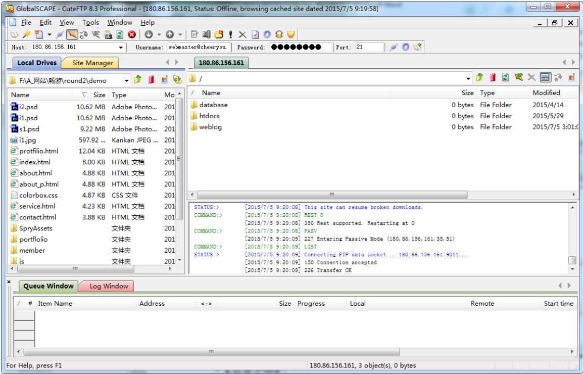
图 7 cuteFTP 界面
