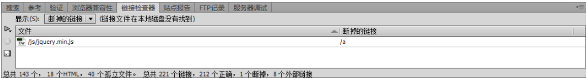
图 3 测试结果
