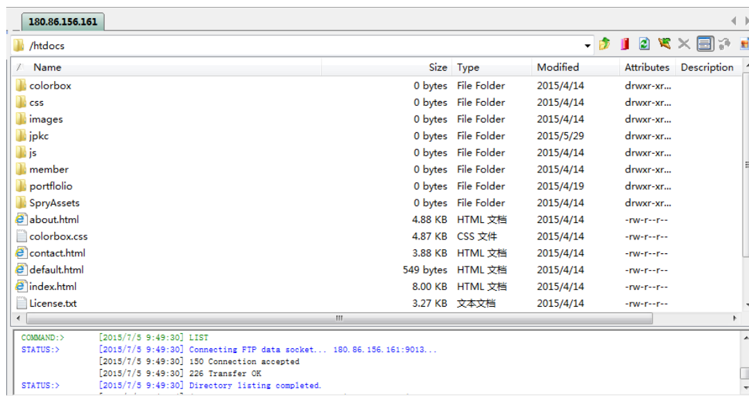
图 8 上传网站
