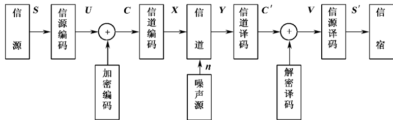
图 1.4 信息传输系统的模型
