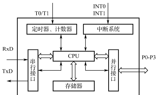
图 1-2 单片机内部结构示意图
