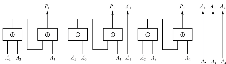
图 3-2-10 海明校验编码逻辑
