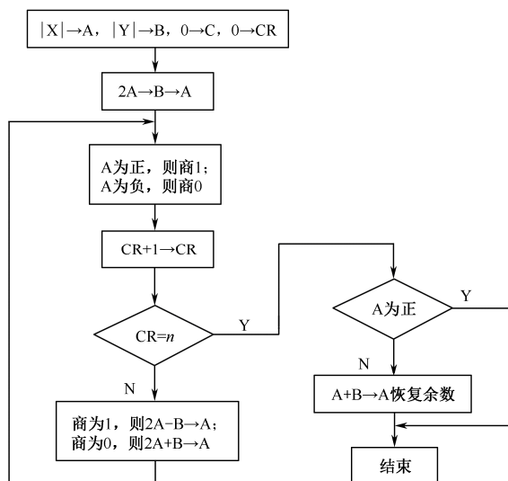
图 3-2-3 原码加减交替除法流程
