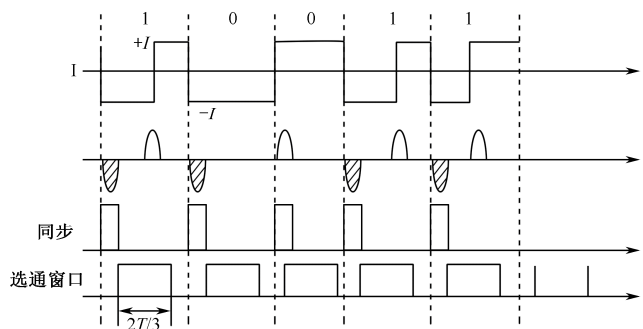
图 3-4-9 FM 制写电流波形
