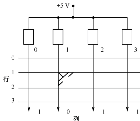
图 3-6-1 一个 4×4 扫描式键盘矩阵
