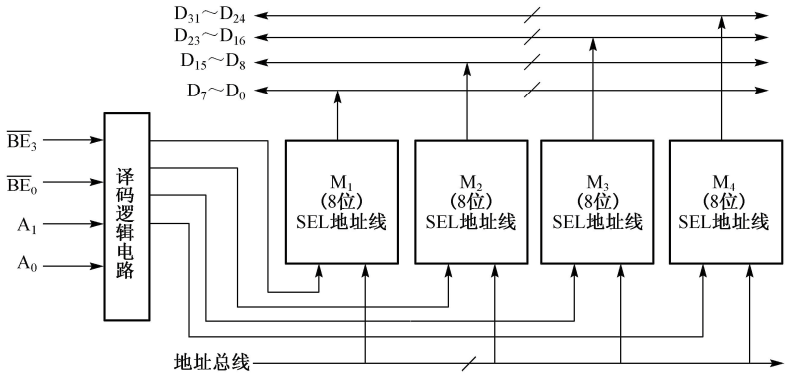
图 3-4-11 存储体连接粗框图
