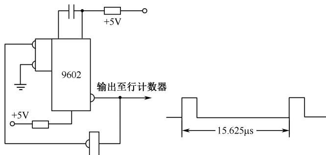
图 3-4-6 动态刷新逻辑
