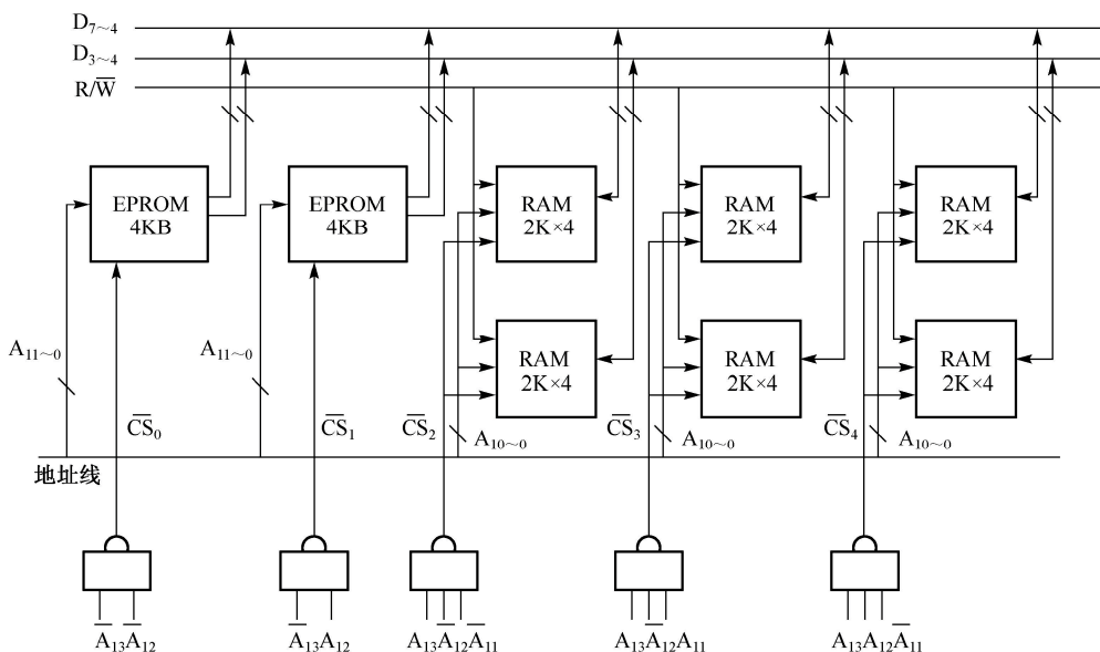
图 3-4-4 逻辑结构图
