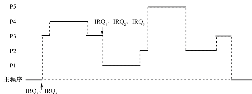
图 3-5-7 CPU 执行中断服务程序的流程
