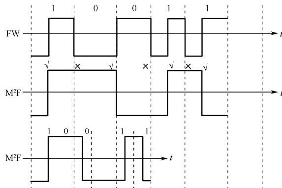
图 3-4-10 M 2 F 制写电流波形
