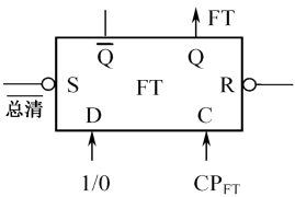
图 3-3-1 取指周期状态触发器
