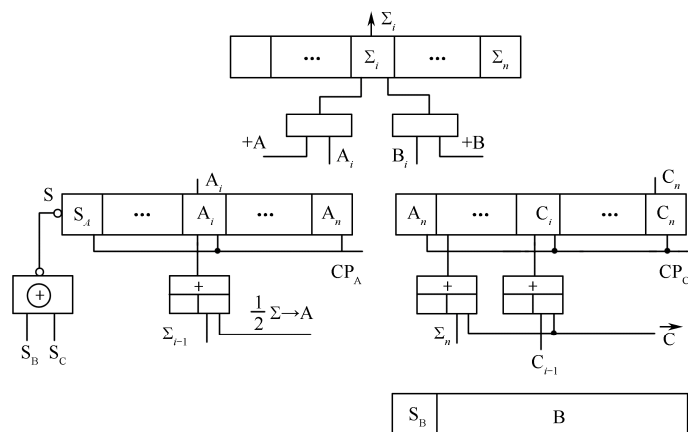
图 3-2-8 原码一位乘法器框图
