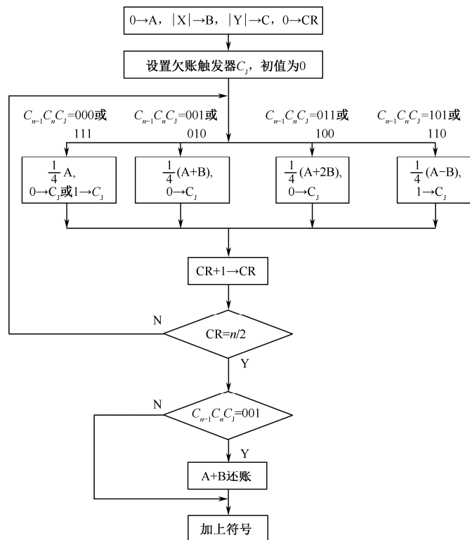
图 3-2-2 原码两位乘法流程
