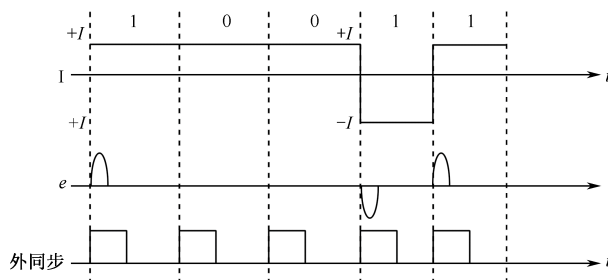
图 3-4-7 NRZ-1 制写电流波形
