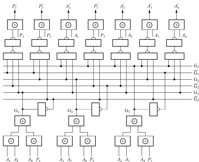
图 3-2-11 海明译码、纠错逻辑
