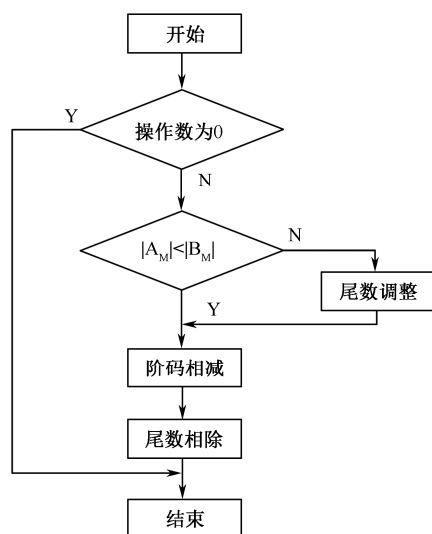
图 3-2-7 浮点除法流程图
