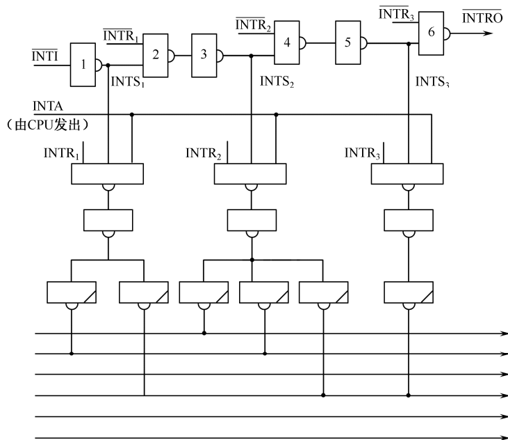
图 3-5-3 多重查询方式判优逻辑图
