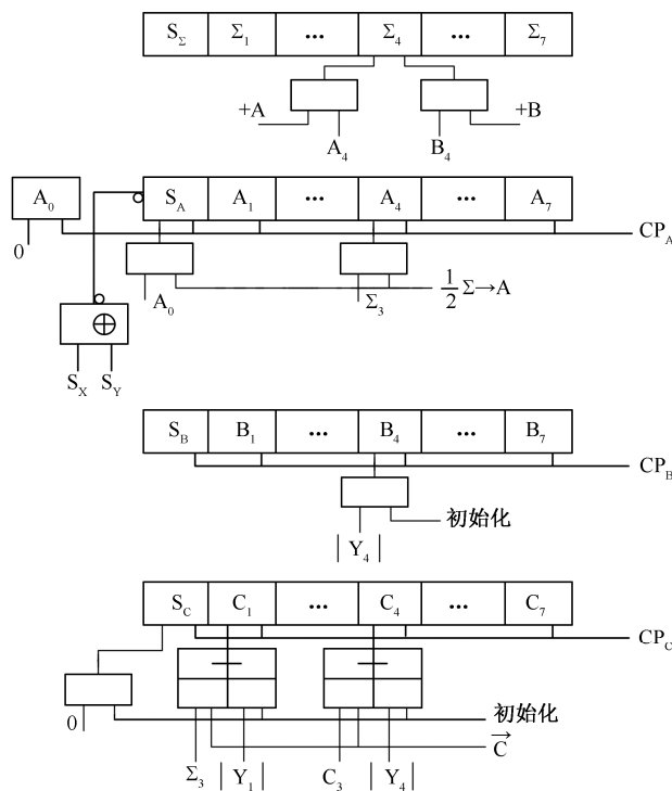
图 3-2-9 乘法器的逻辑图
