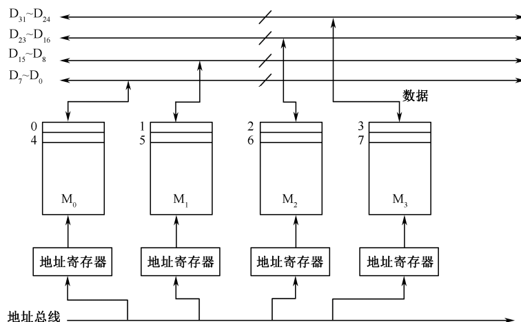
图 3-4-12 多体交叉存储器与系统总线连接方式
