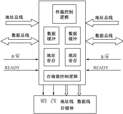
图 3-4-15 以常规存储芯片构成双端口存储器逻辑
