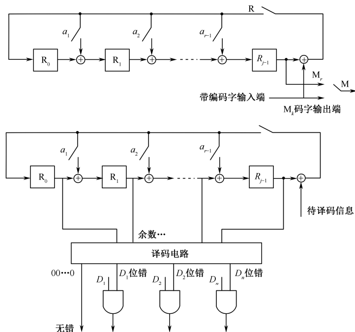
图 3-2-13 循环校验码的编码、译码、校正电路
