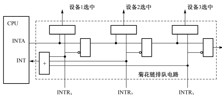
图 3-5-4 菊花链式判优逻辑图
