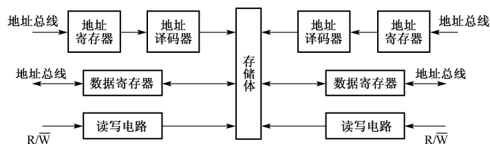
图 3-4-14 双 CPU 共享存储器连接图
