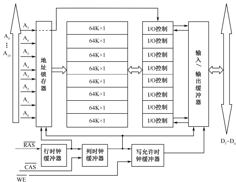
图 3-4-5 存储器连接逻辑图
