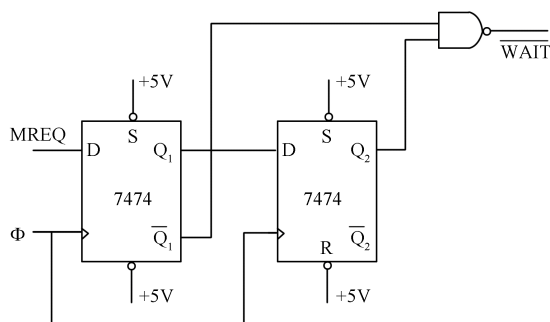
图 3-4-13 产生等待状态 READY 信号的逻辑
