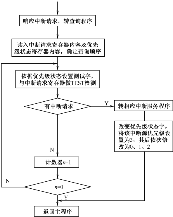
图 3-5-2 轮流优先级流程图
