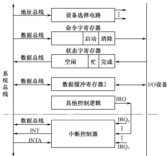
图 3-5-5 中断接口逻辑图
