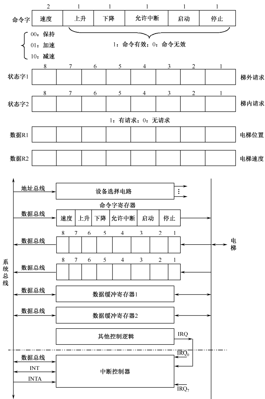
图 3-5-6 用于电梯控制的命令字状态字格式
