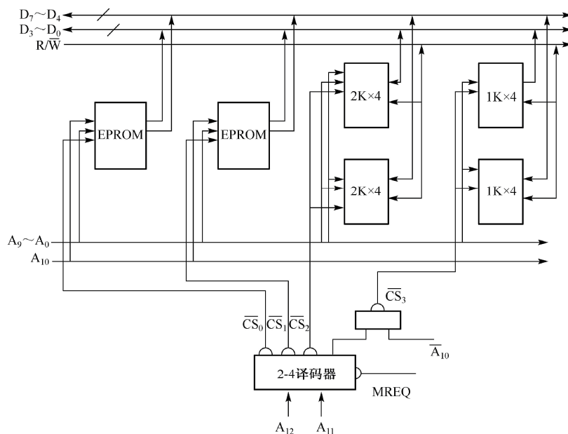
图 3-4-2 存储器逻辑图
