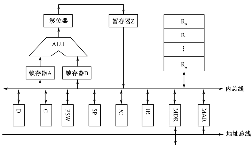
图 3-3-3 新设计的模型机
