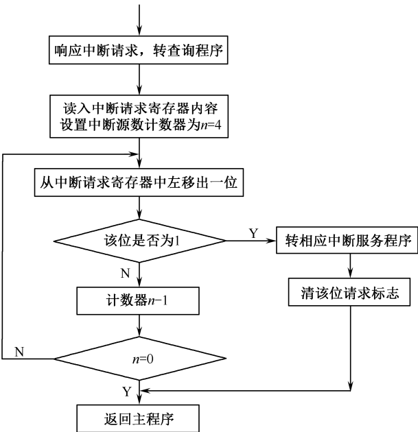
图 3-5-1 固定优先级流程图
