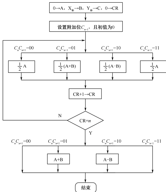
图 3-2-1 补码一位乘法流程
