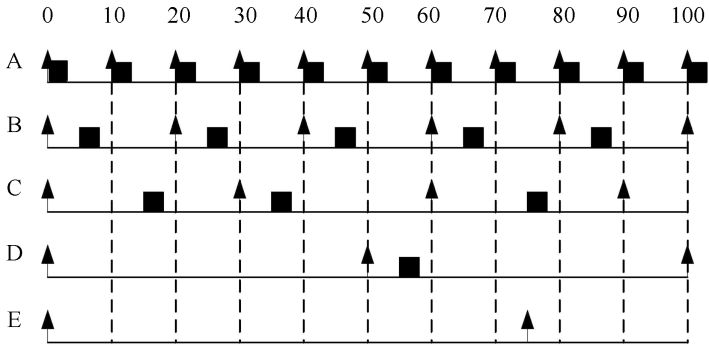
图 3-5-8 通道相应时间关系
