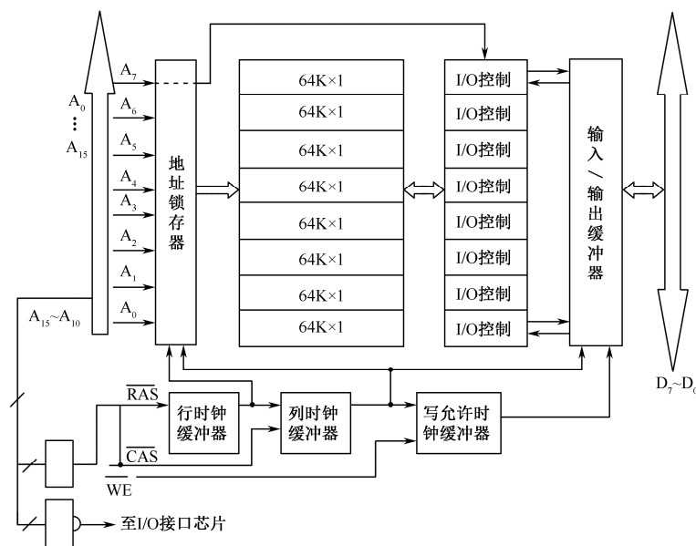
图 3-4-3 存储器逻辑图
