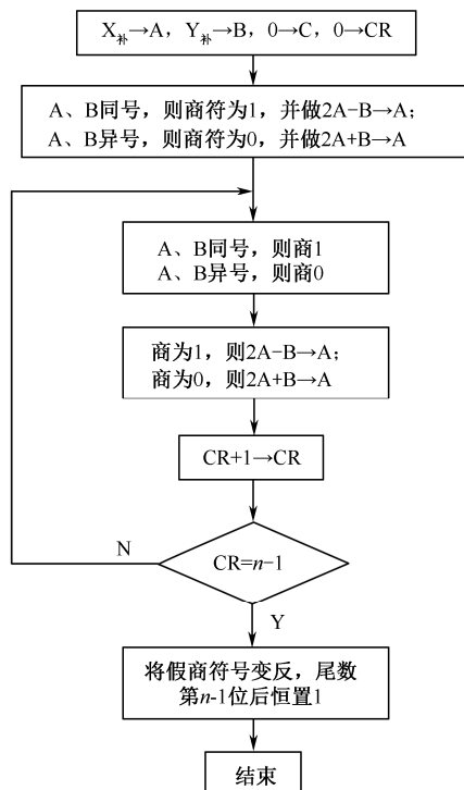
图 3-2-4 补码加减交替除法流程图
