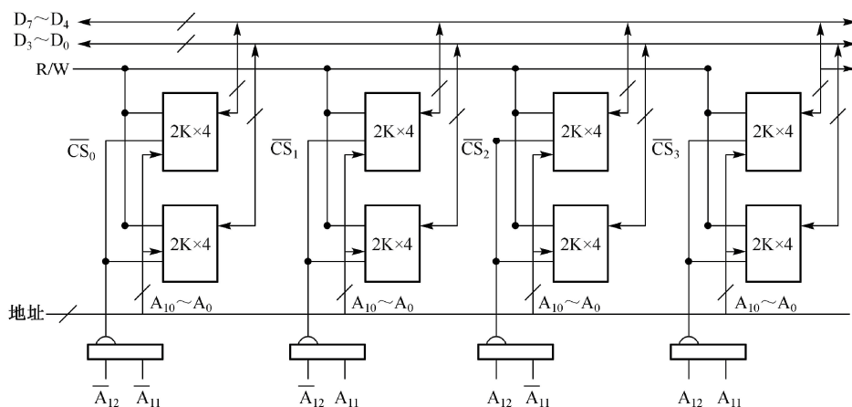
图 3-4-1 存储器逻辑图
