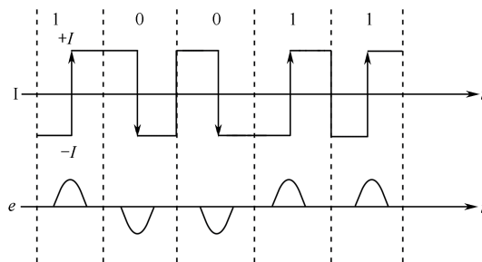
图 3-4-8 调相制写电流波形
