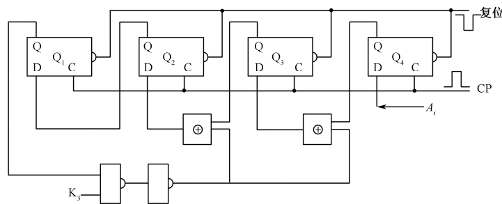
图 3-2-12 模 2 除法器的逻辑结构图
