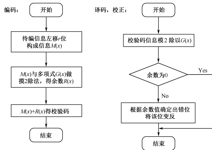
图 3-2-14 循环校验码的编码、译码、校正子程序流程
