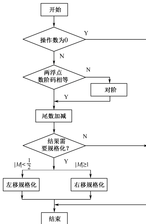
图 3-2-5 浮点加减流程图
