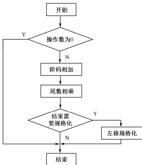
图 3-2-6 浮点乘法流程图
